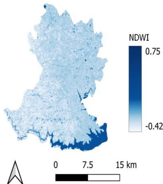
Fig. 4. NDWI Map
