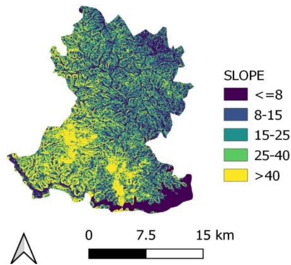
Fig. 7. Slope Map
