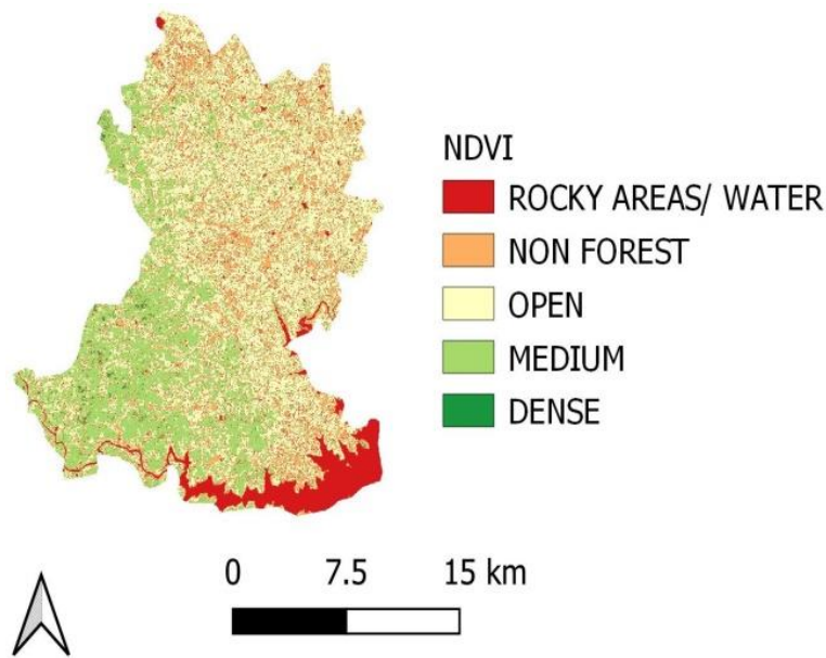
Fig. 3. NDVI Map
